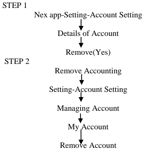
Fig 4.Nex Spy
